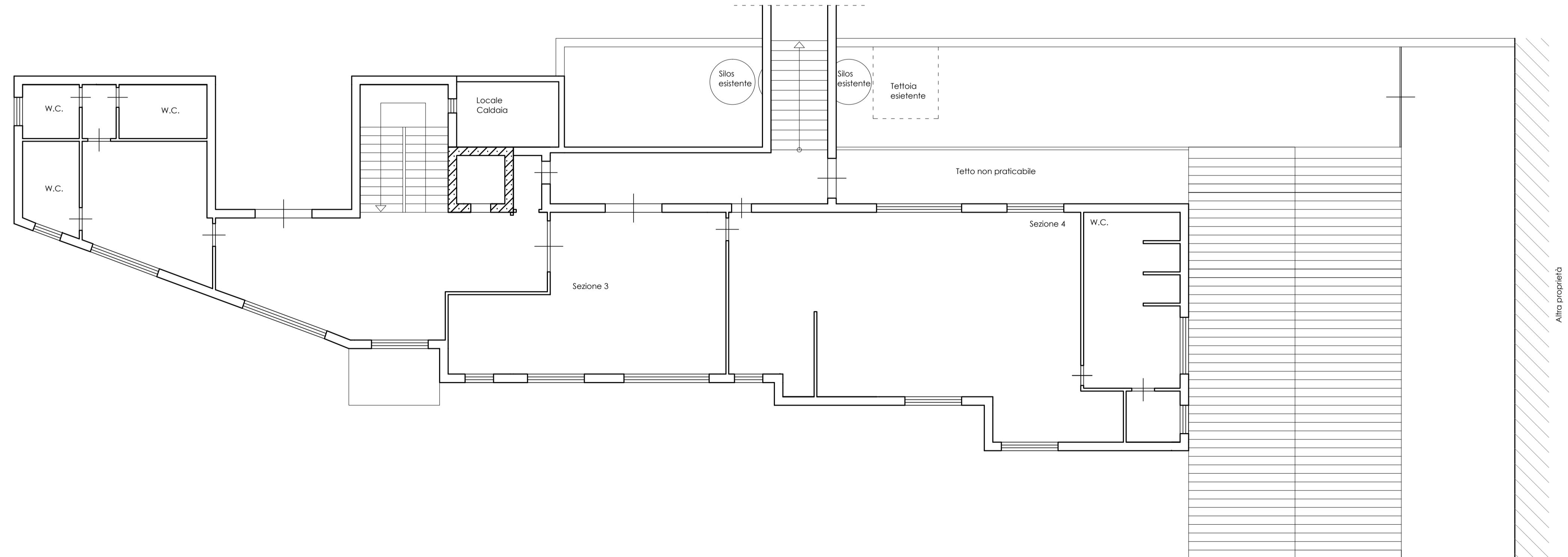
Pianta piano primo scala 1:100
