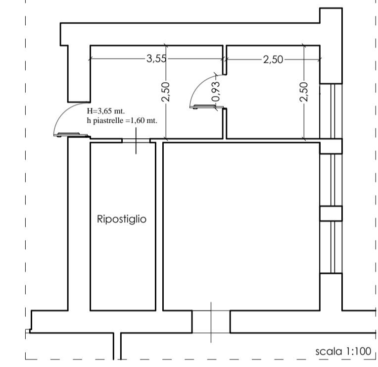
Particolare 1 - Progetto
